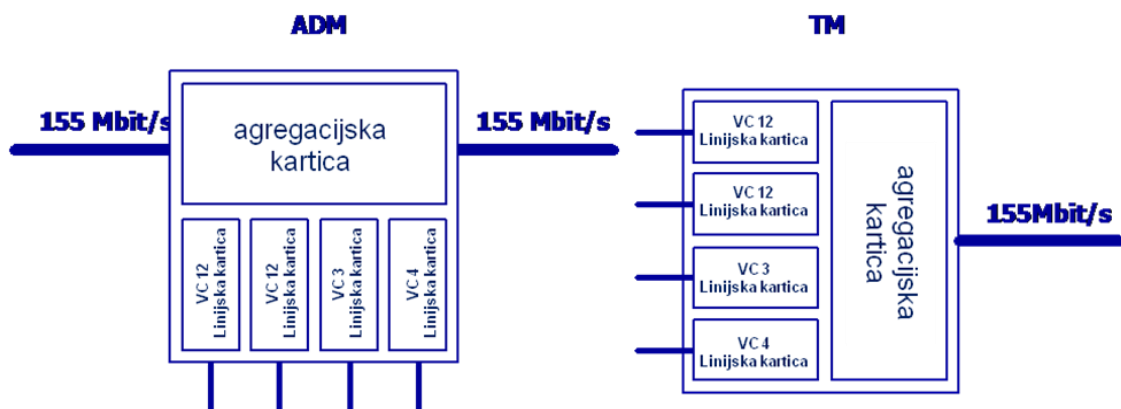
Slika 12.1 STM-1
